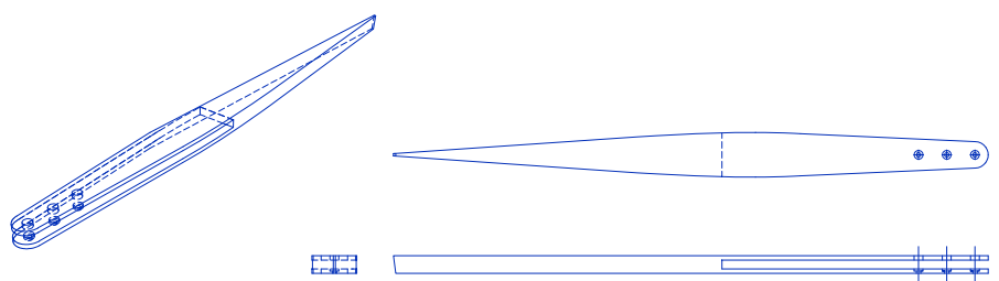
BOOM
