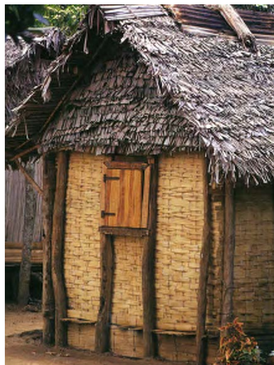
Ci-dessous : Maison à Madagascar reposant sur une fondation en terre maintenue par un coffrage en planches de bambou. Sol recouvert de planches de bambou, mur en tressage de lattes de bambou. Le faitage de toiture porte la marque des modernisations successives : lattes de bambou recouvertes de tôle ondulée, elle-même maintenue par un chaume.
