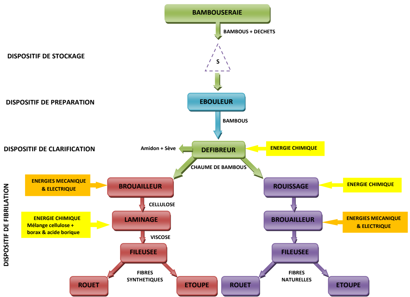
LES DEUX PROCEDES DE FABRICATION DE TEXTILE A PARTIR DU BAMBOU.
