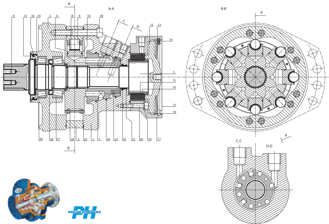
FIGURE 2.3 – Moteur hydraulique Poclain
