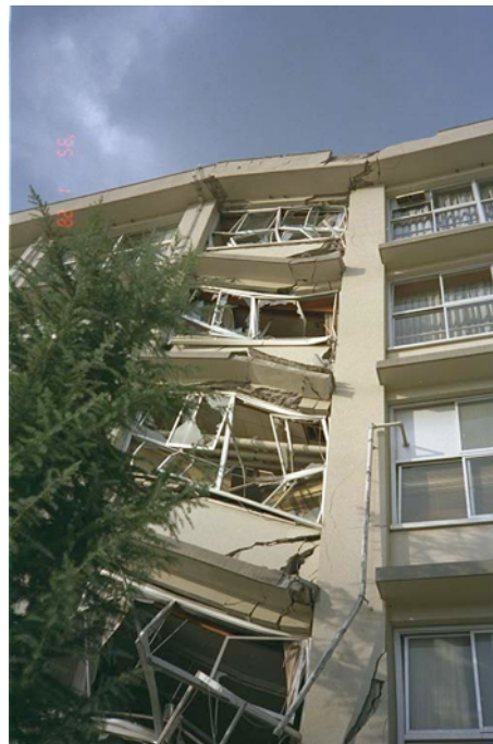
FIGURE 7.2 – Collision entre étages
