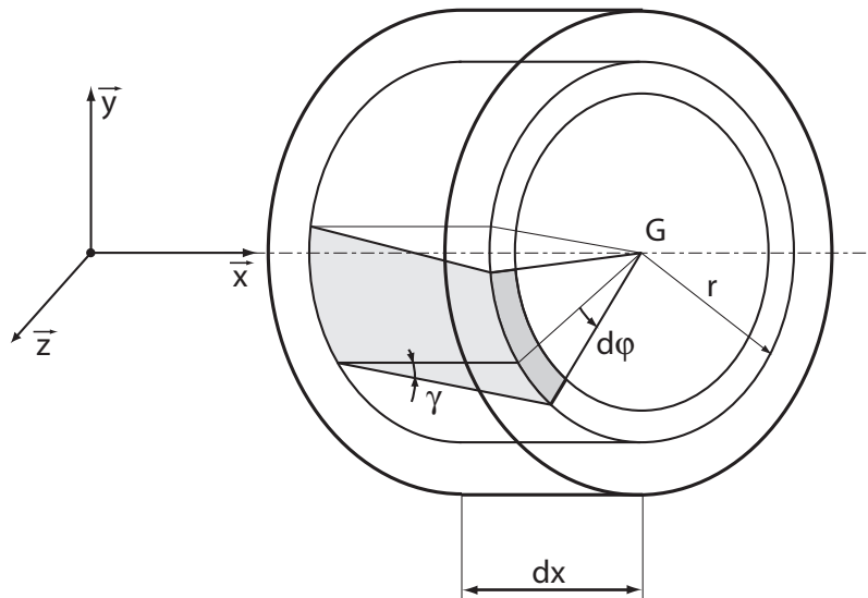
FIGURE 4.5 – Isolement d'un disque de longueur dx
