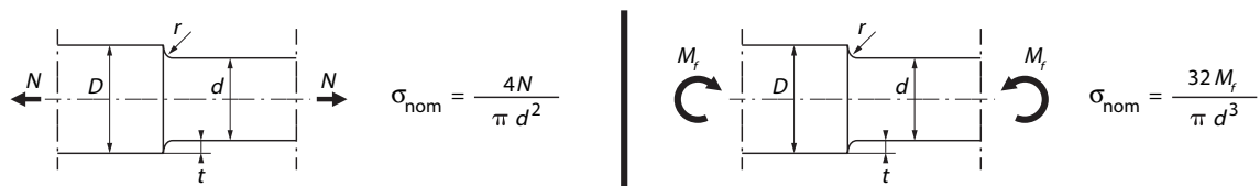
FIGURE 6.6 – Calcul de la contrainte nominale
