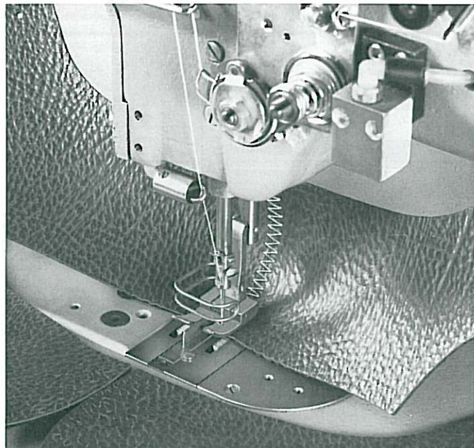
Adler 98-FAP-2-8 und Spezialgarnitur F 224, stumpfes Zusammenstoßen der Quartiere and special sewing components F 224 for butt-joining quarters avec jeu de pièces de couture spécial F 224 pour l'assemblage bout à bout des liges y juego de costura especial F 224 para unir a tope los talones
